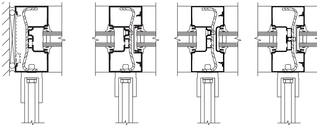
TRIFAB® VG 451T JAMB (TF VG 451 & 451UT SIMILAR)
