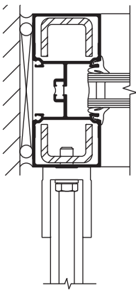
TRIFAB® VG 451T JAMB (TF VG 451 SIMILAR)
